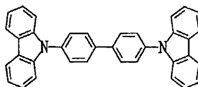
CBP
