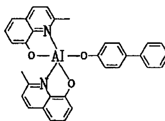
BAlq
